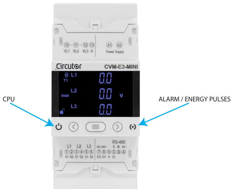
Figura 27: Indicadores LED del CVM-E3-MINI.
