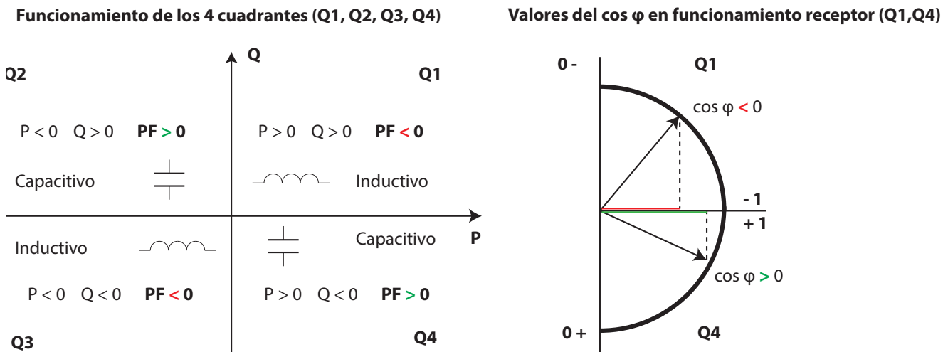
Figura 25: Convenio de medida IEEE.
