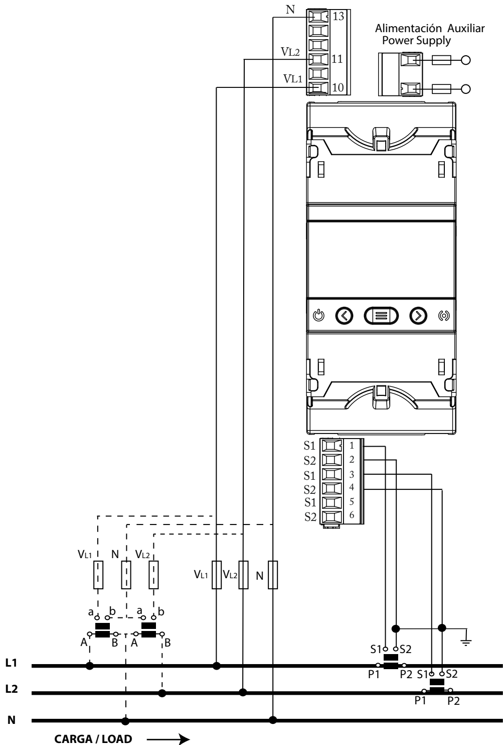
Figura 14: Medida bifásica con conexión a 3 hilos: CVM-E3-MINI-ITF y CVM-E3-MINI-ITF-WiEth.
