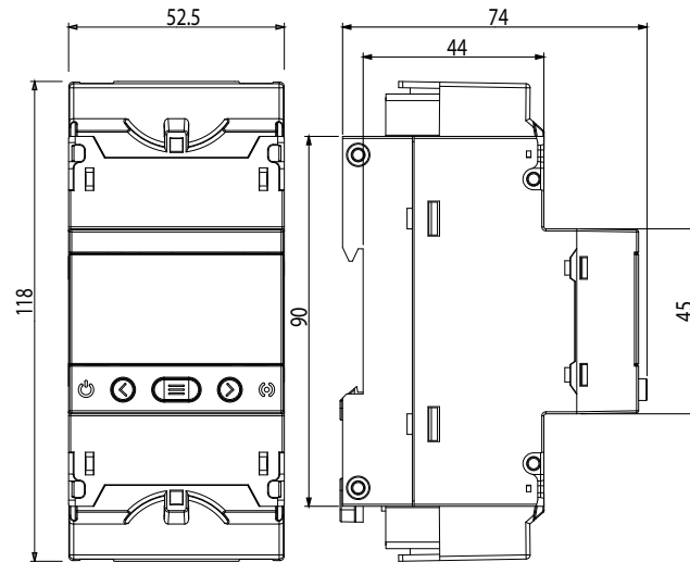
Figura 37: Dimensiones del CVM-E3-MINI.
