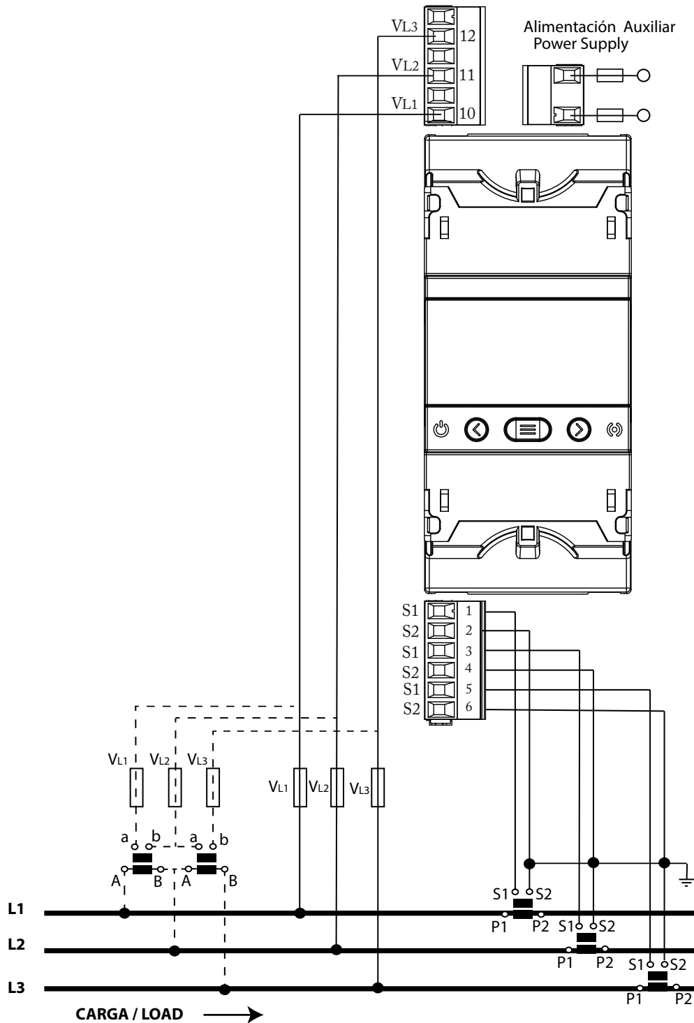
Figura 9: Medida trifásica con conexión a 3 hilos: CVM-E3-MINI-ITF y CVM-E3-MINI-ITF-WiEth.
