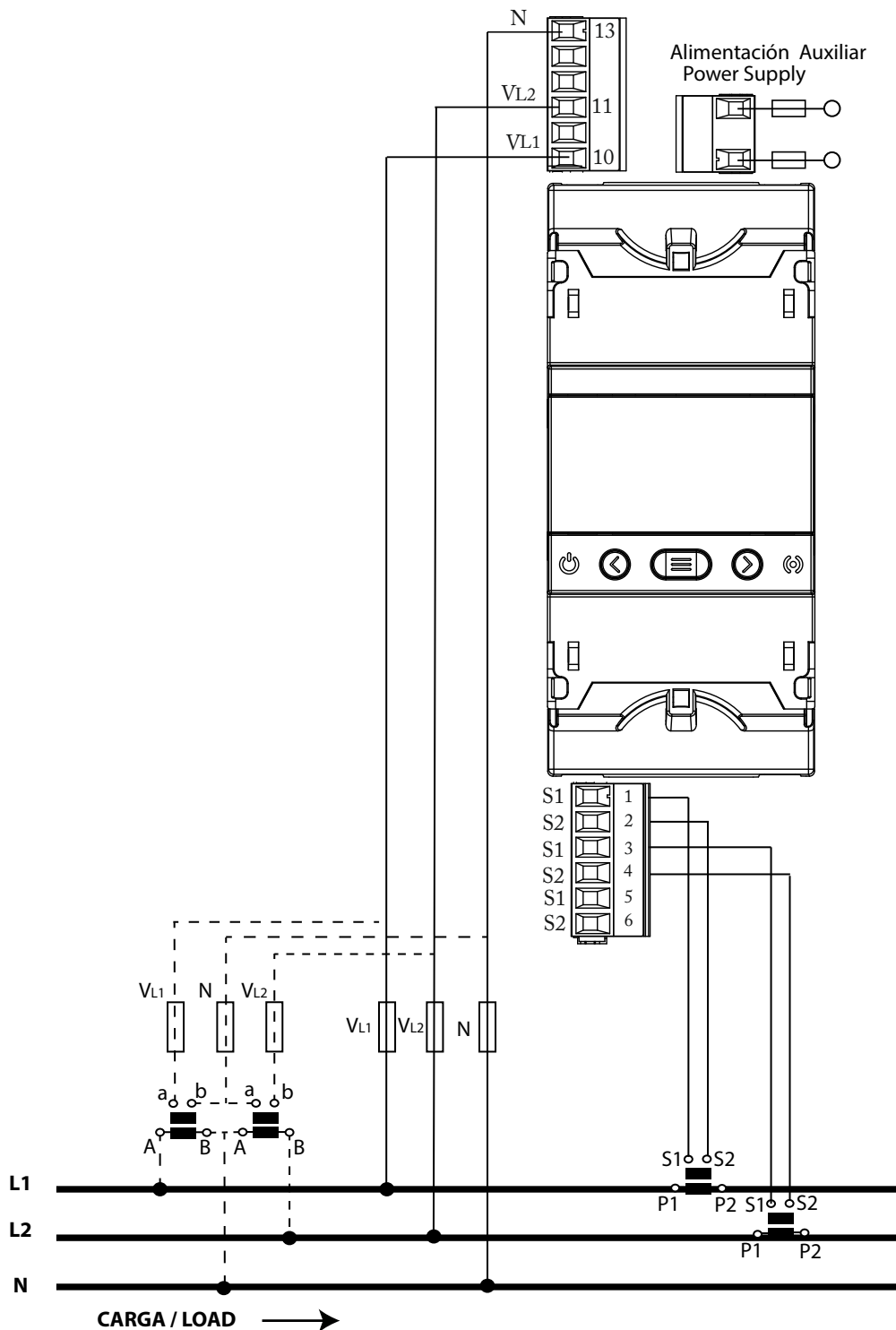
Figura 15: Medida bifásica con conexión a 3 hilos: CVM-E3-MINI-MC y CVM-E3-MINI-MC-WiEth.
