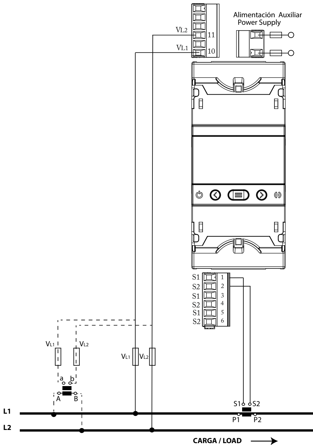
Figura 18: Medida monofásica de fase a fase de 2 hilos: CVM-E3-MINI-MC y CVM-E3-MINI-MC-WiEth.
