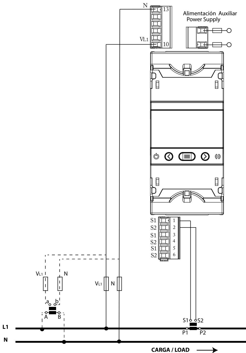
Figura 21: Medida monofásica de fase a neutro de 2 hilos: CVM-E3-MINI-MC y CVM-E3-MINI-MC-WiEth.
