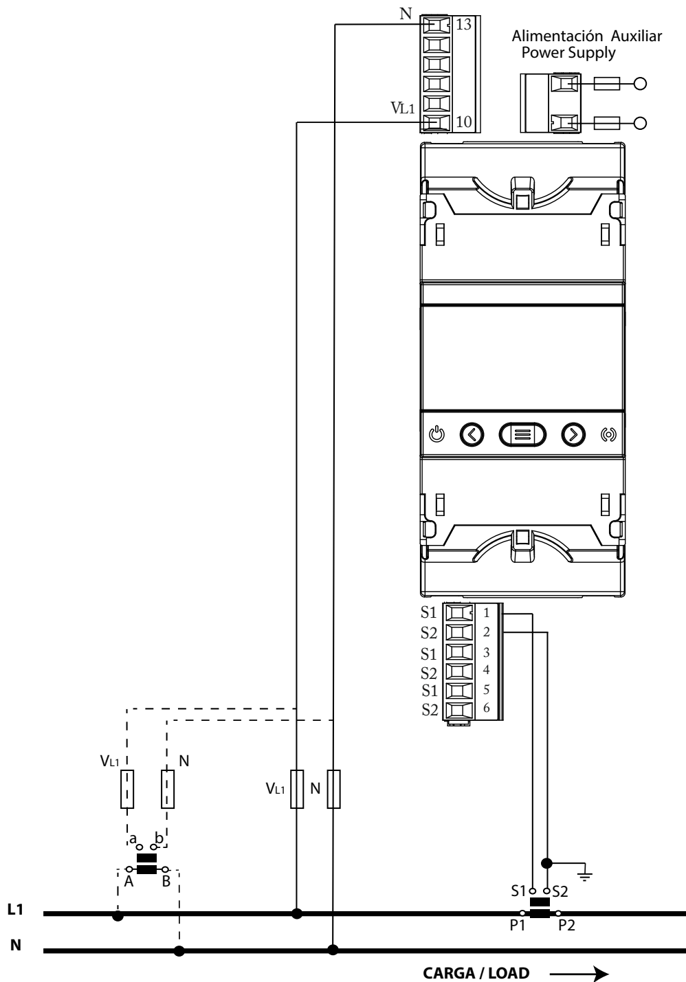
Figura 20: Medida monofásica de fase a neutro de 2 hilos: CVM-E3-MINI-ITF y CVM-E3-MINI-ITF-WiEth.
