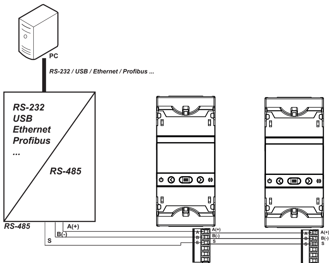
Figura 33: Esquema de conexionado RS-485.
