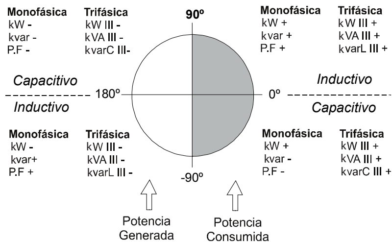
Figura 23: Convenio de medida CIRCUITOR.
