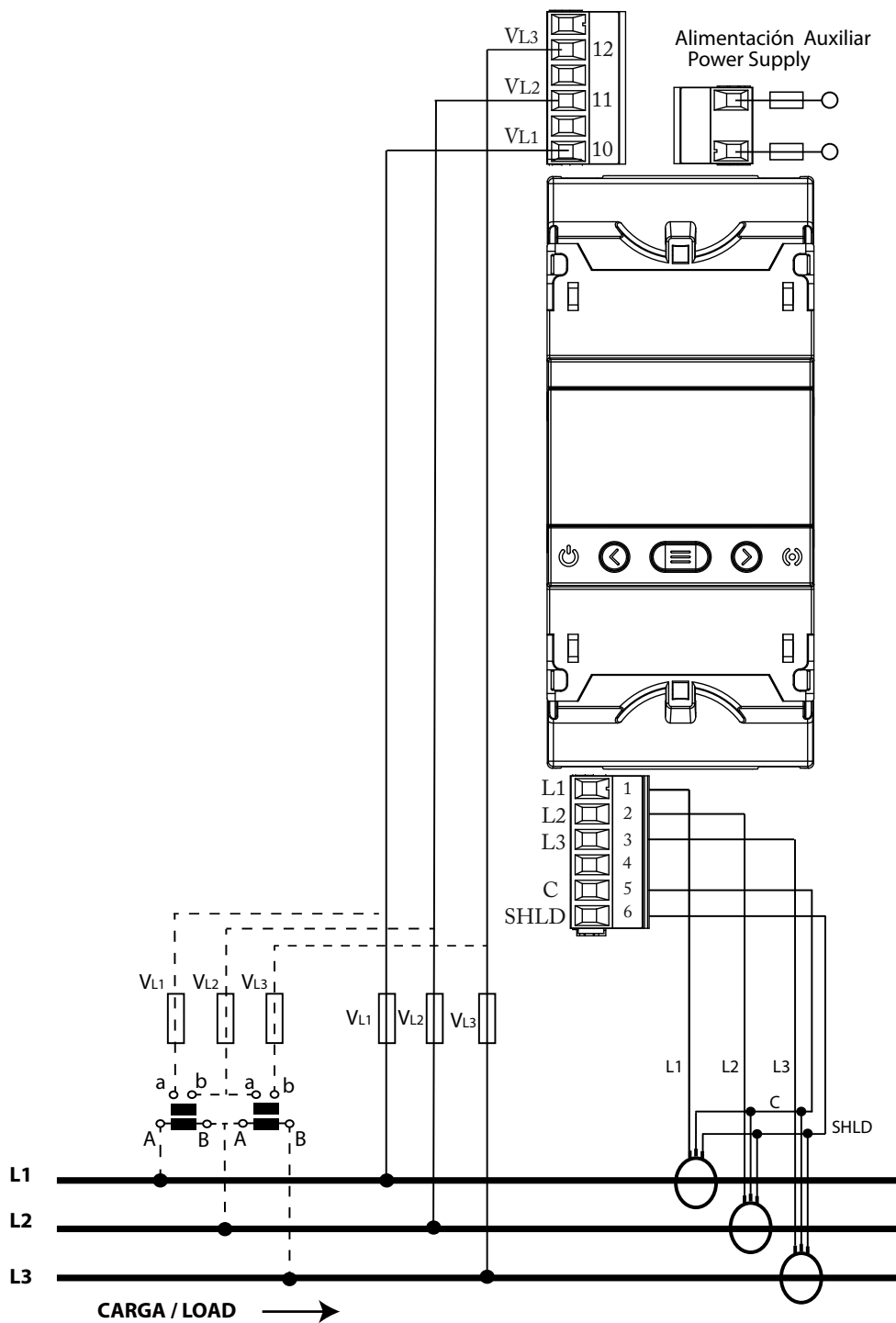
Figura 11: Medida trifásica con conexión a 3 hilos: CVM-E3-MINI-FLEX y CVM-E3-MINI-FLEX-WiEth.
