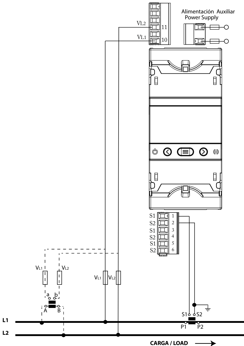
Figura 17: Medida monofásica de fase a fase de 2 hilos: CVM-E3-MINI-ITF y CVM-E3-MINI-ITF-WiEth.
