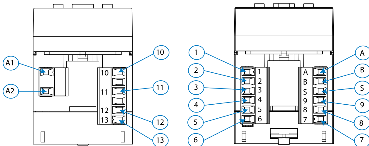
Figura 4: Bornes del CVM-E3-MINI-ITF / -MC / -FLEX: Superior - Inferior.
