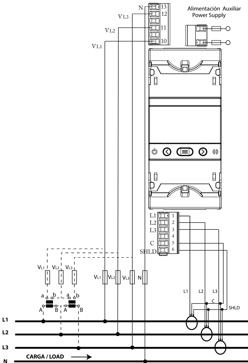
Figura 8: Medida trifásica con conexión a 4 hilos: CVM-E3-MINI-FLEX y CVM-E3-MINI-FLEX-WiEth.
