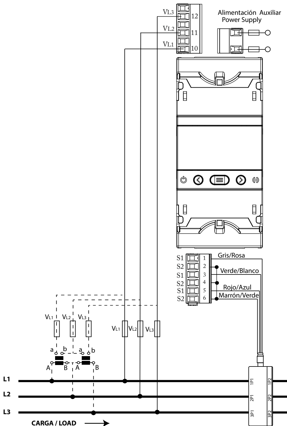
Figura 10: Medida trifásica con conexión a 3 hilos: CVM-E3-MINI-MC y CVM-E3-MINI-MC-WiEth.
