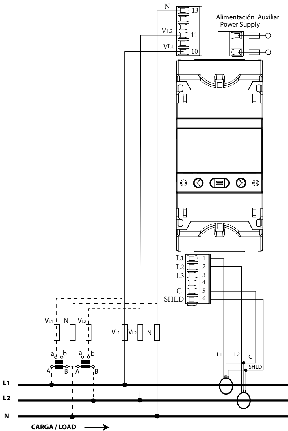
Figura 16: Medida bifásica con conexión a 3 hilos: CVM-E3-MINI-FLEX y CVM-E3-MINI-FLEX-WiEth.
