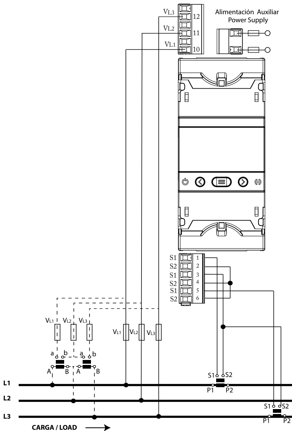
Figura 13: Medida trifásica con conexión a 3 hilos y transformadores en conexión ARON: CVM-E3-MINI-MC y CVM-E3-MINI-MC-WiEth.
