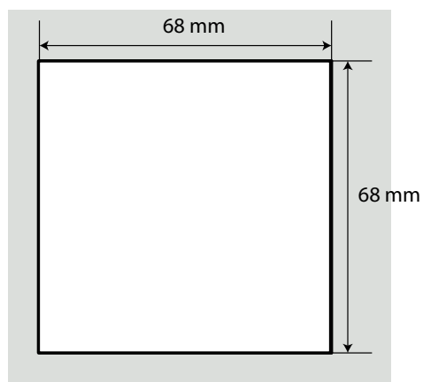
Figura 3: Corte de panel.
