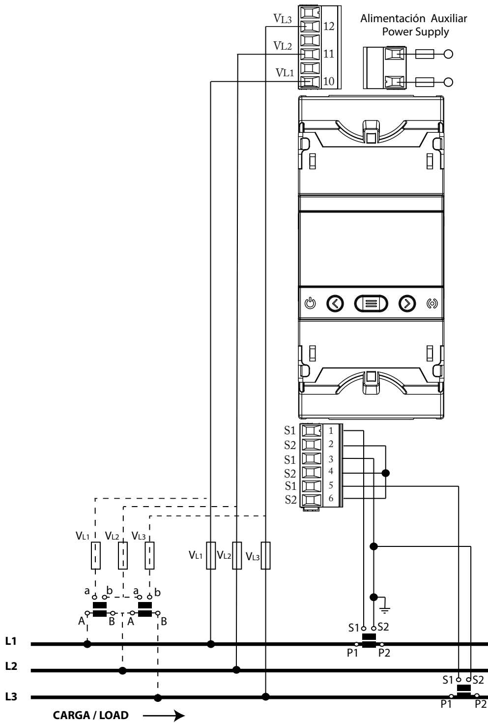
Figura 12: Medida trifásica con conexión a 3 hilos y transformadores en conexión ARON: CVM-E3-MINI-ITF y CVM-E3-MINI-ITF-WiEth.
