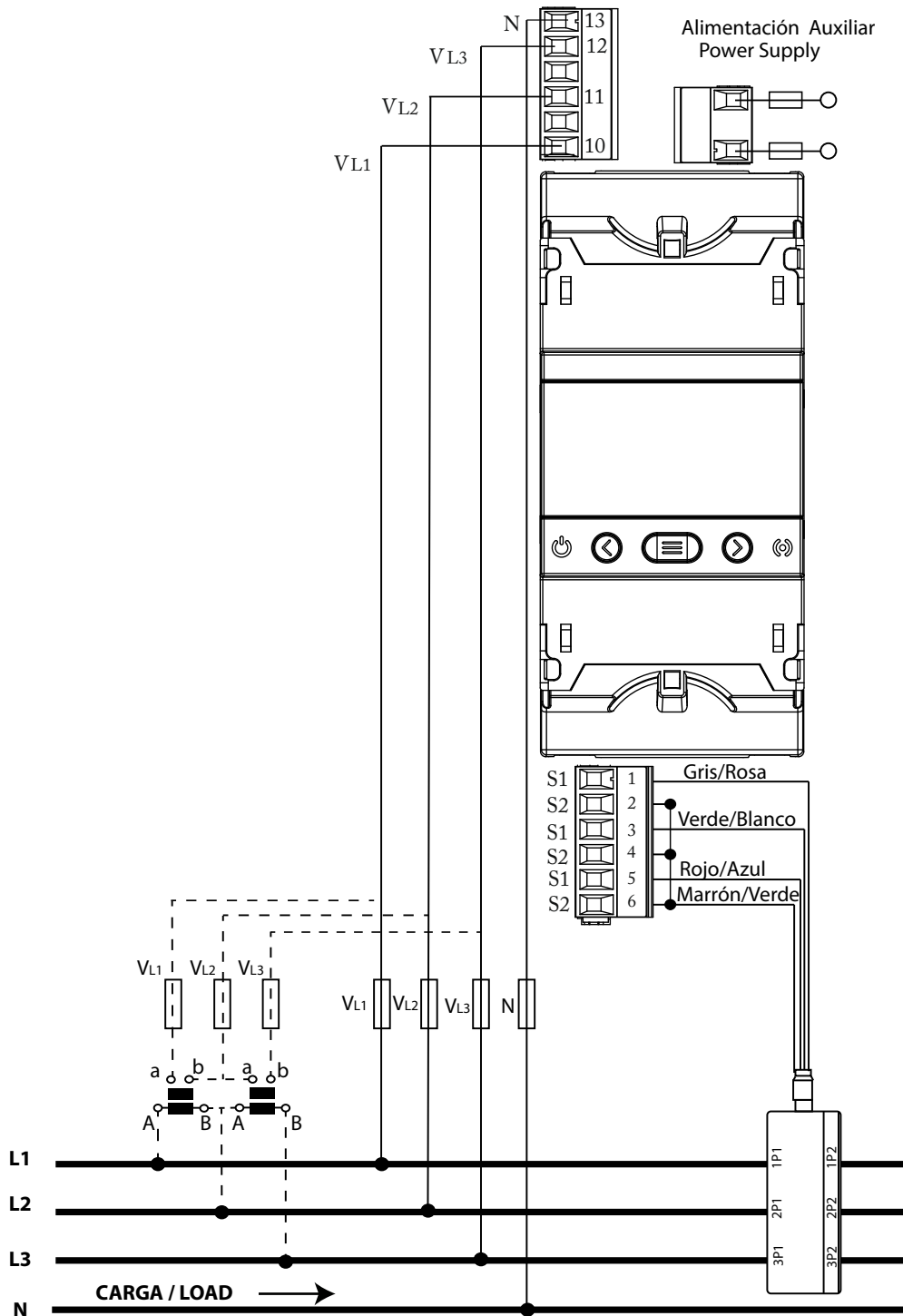
Figura 7: Medida trifásica con conexión a 4 hilos: CVM-E3-MINI-MC y CVM-E3-MINI-MC-WiEth.
