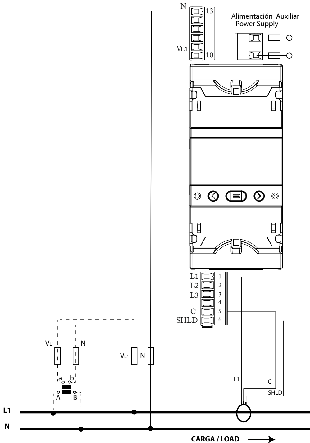
Figura 22: Medida monofásica de fase a neutro de 2 hilos: CVM-E3-MINI-FLEX y CVM-E3-MINI-FLEX-WiEth.
