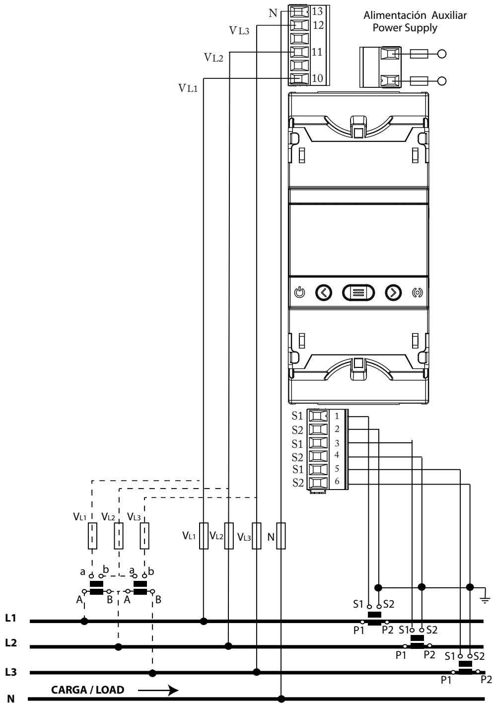
Figura 6: Medida trifásica con conexión a 4 hilos: CVM-E3-MINI-ITF y CVM-E3-MINI-ITF-WiEth.
