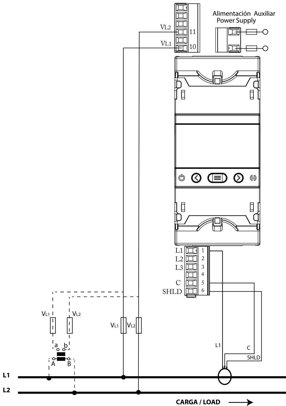
Figura 19: Medida monofásica de fase a fase de 2 hilos: CVM-E3-MINI-FLEX y CVM-E3-MINI-FLEX-WiEth.
