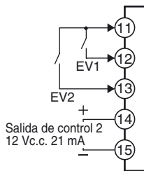
E53-CNQFN2
