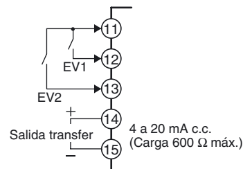
E53-CN01N2
